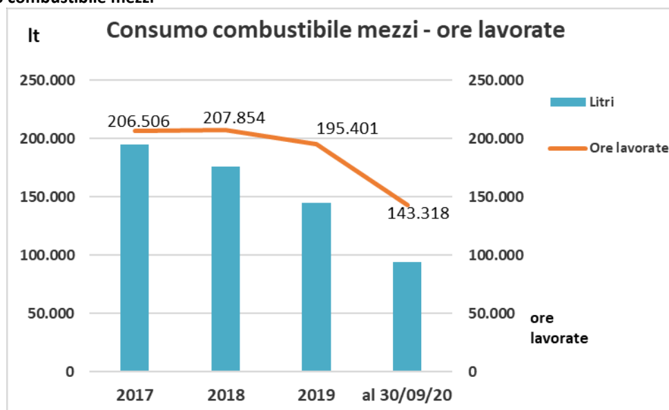
Fig. 13 - Consumo combustibile mezzi
