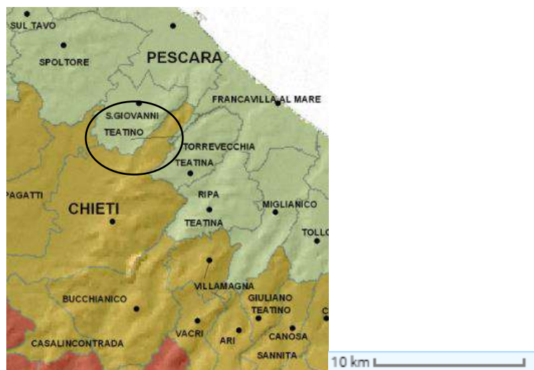
Fig. 7 – Suddivisione zone sismiche
